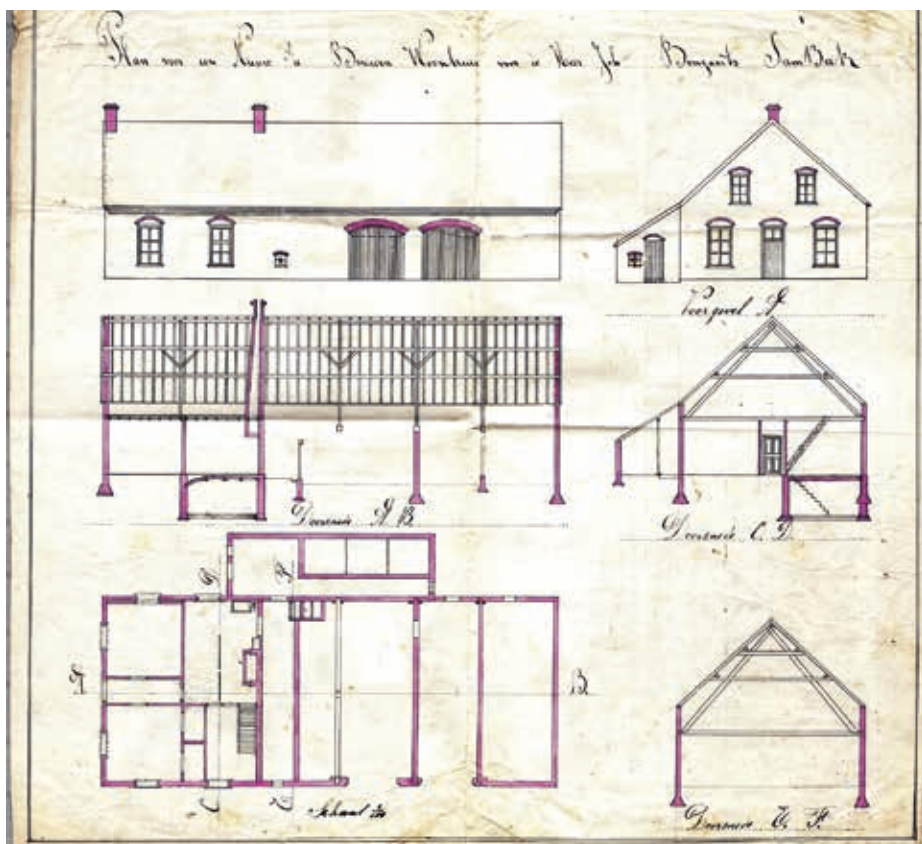
Bouwtekening van de Sambeekse aannemer Hendrikus Kerstjens van het huidige pand Hoogeindseweg 6 + 6b.
